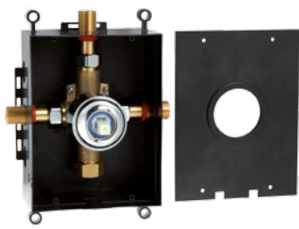
Montážní box s podomítkovou baterií Montážny box s podomietkovou batériou
